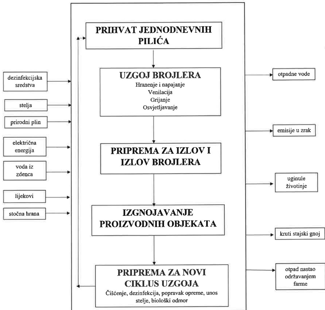
Prilog 2. Bok dijagram tehnološkog procesa na postojećem postrojenju za intenzivan uzgoj peradi Farma 8
